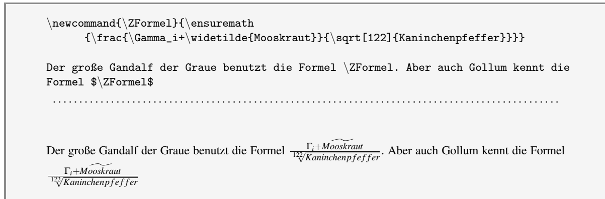
Abbildung 26: Ein Makro für den Mathematik-Modus
